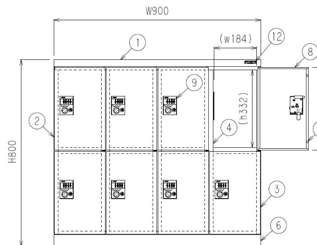
多目的ロッカー 4列2段
