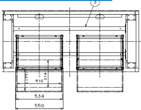
イトラム 引出付きテーブル仕様
