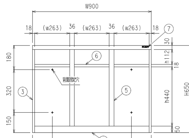
オープンシューズボックス 3列1段
